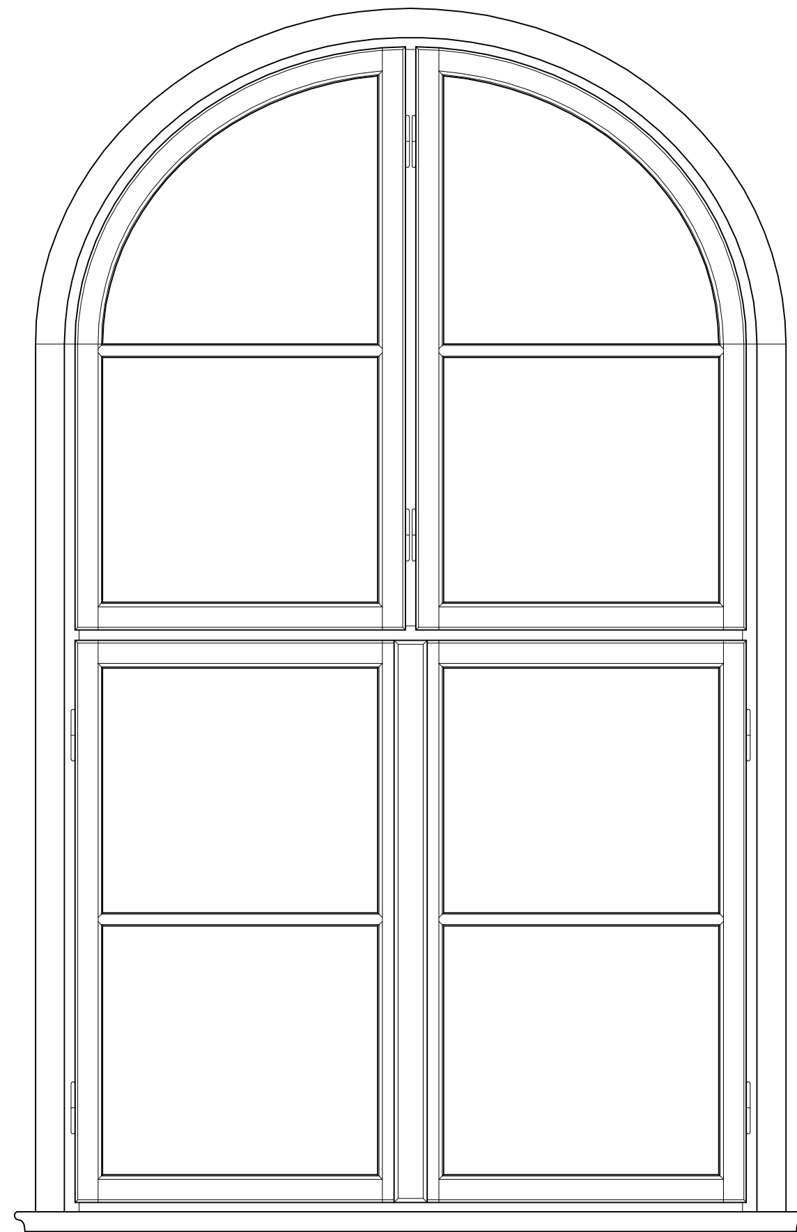
Okno typu D i D1 rekonstrukcja oryginalnego okna skala 1:10
